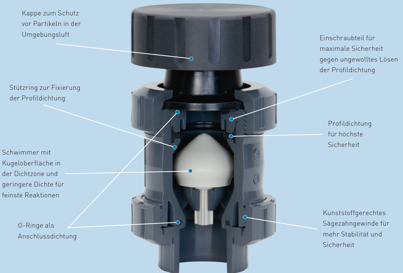
Belüftungs- und Entlüftungsventil Typ 591: ohne Feder (Abbildung oben) Belüftungsventil Typ 595: mit Feder
