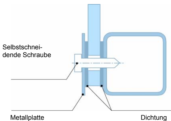
Abb. 4 : Mechanische Befestigung
