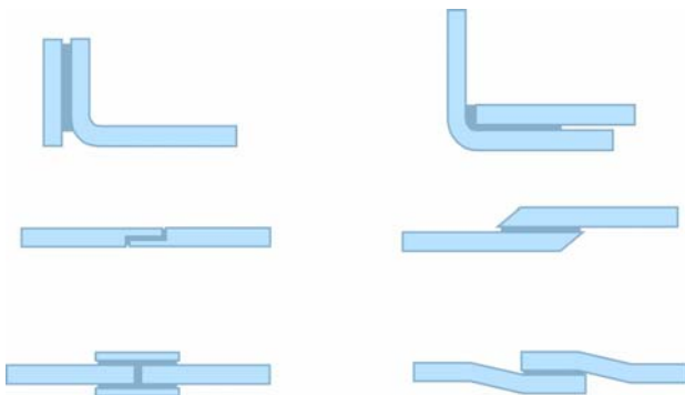
Abb. 1: Verschiedene Klebeverbindungen.
